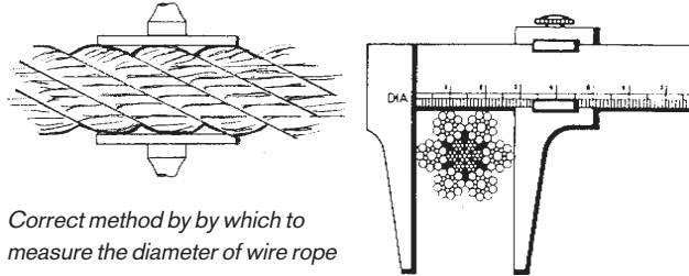
Fig 3. Wire rope
